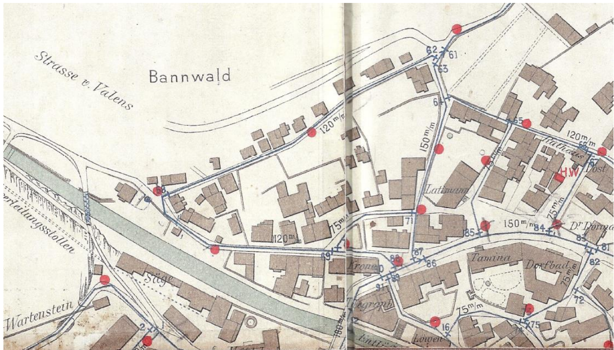
Hydrantennetz 1899 (Quelle: IG Sprützhüsli)
