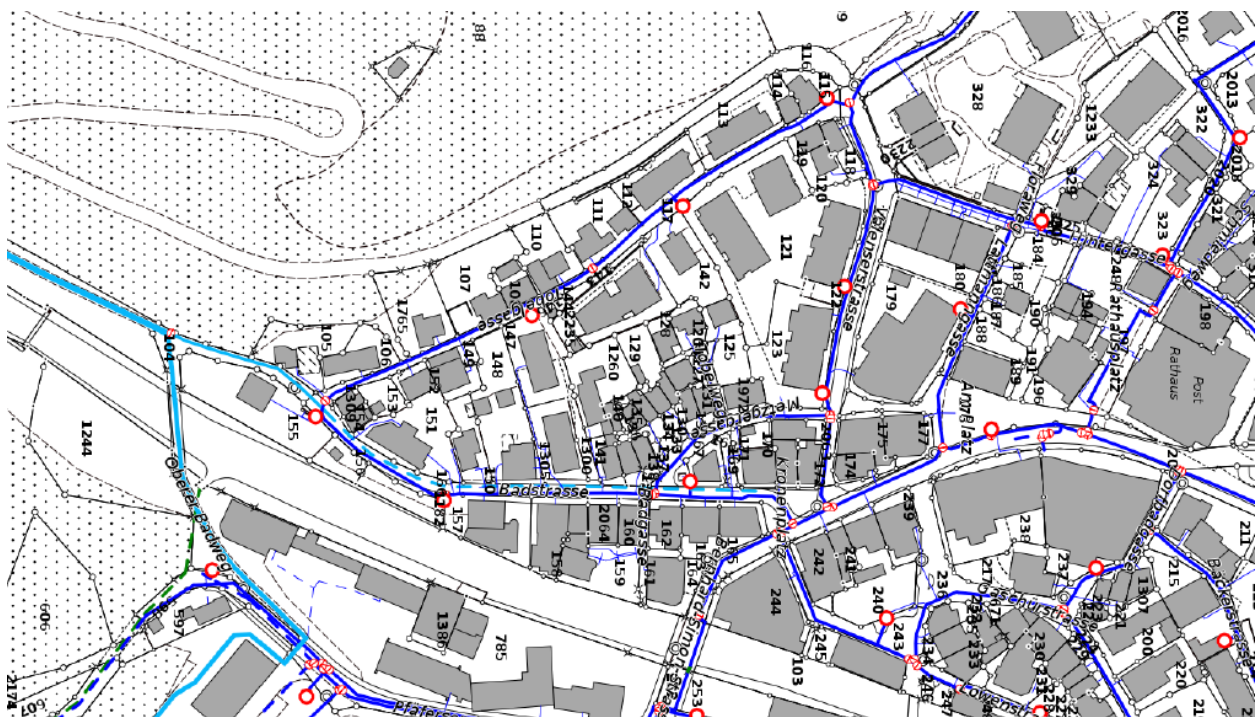
Wasserversorgung 2021 (Quelle: WEB-GIS Bad Ragaz)
